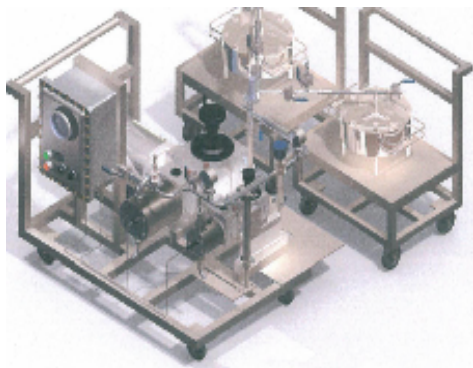
脂质体量产设备 效果图
